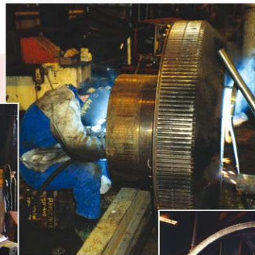
▼ Rechargement d'un moyeu d'embrayage
