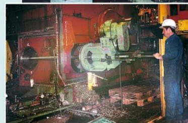
▲ Alésage portée de ligne d'arbre sur presse horizontale
